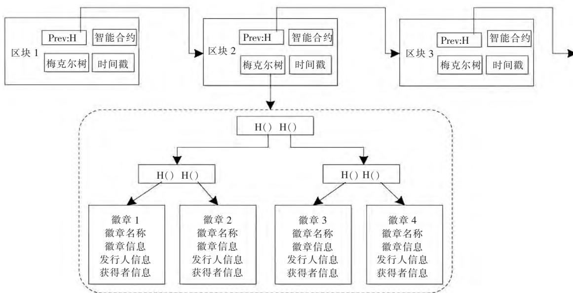
图 12 开放徽章区块链原理
